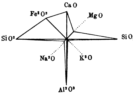
Fig. 2. Melaphyr von der Decke westlich von Cadin brut 2300 m (PROBOSCHT analys.).
